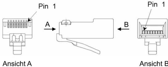
Pin-Nummerierung RJ45-Stecker
